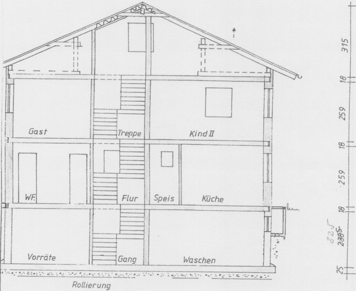
Schnitt A-A
